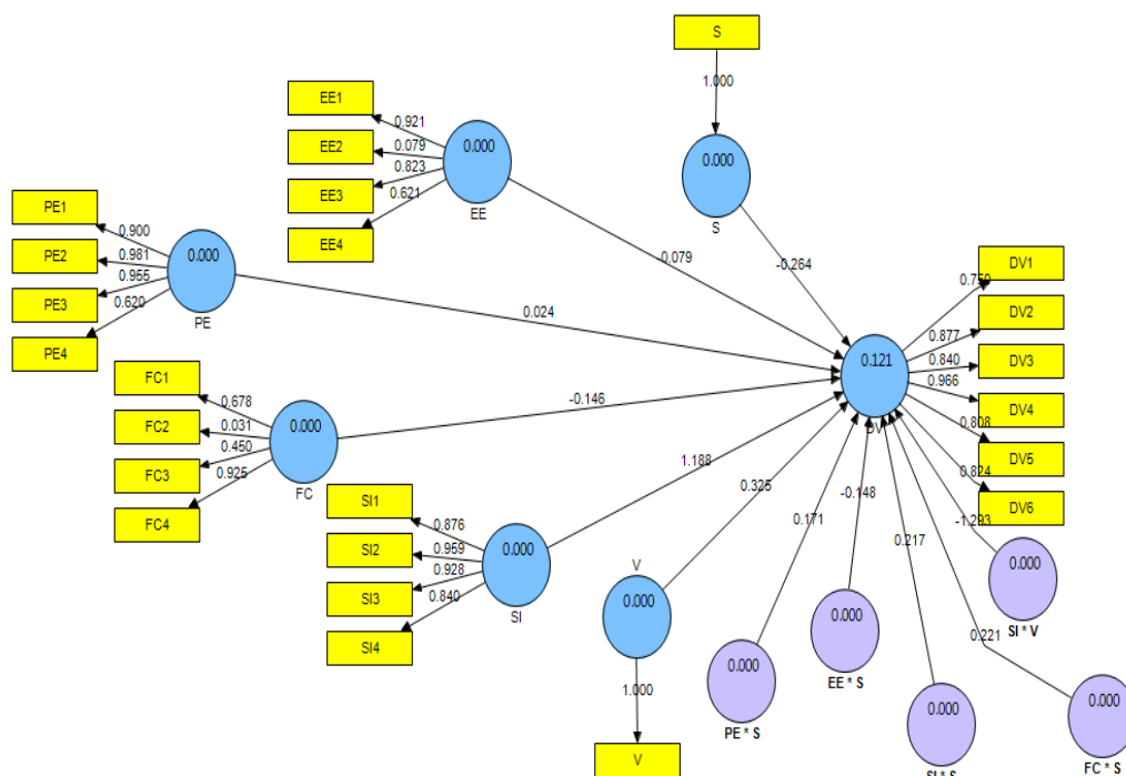
شکل ۲- معیار ضریب معناداری Z
