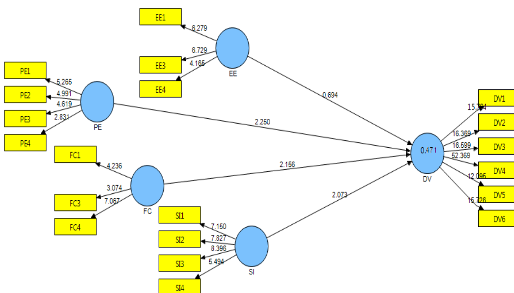
شکل ۳- معيار ضريب معناداري Z بعد از حذف اثر متغيرهاي تعديلی
